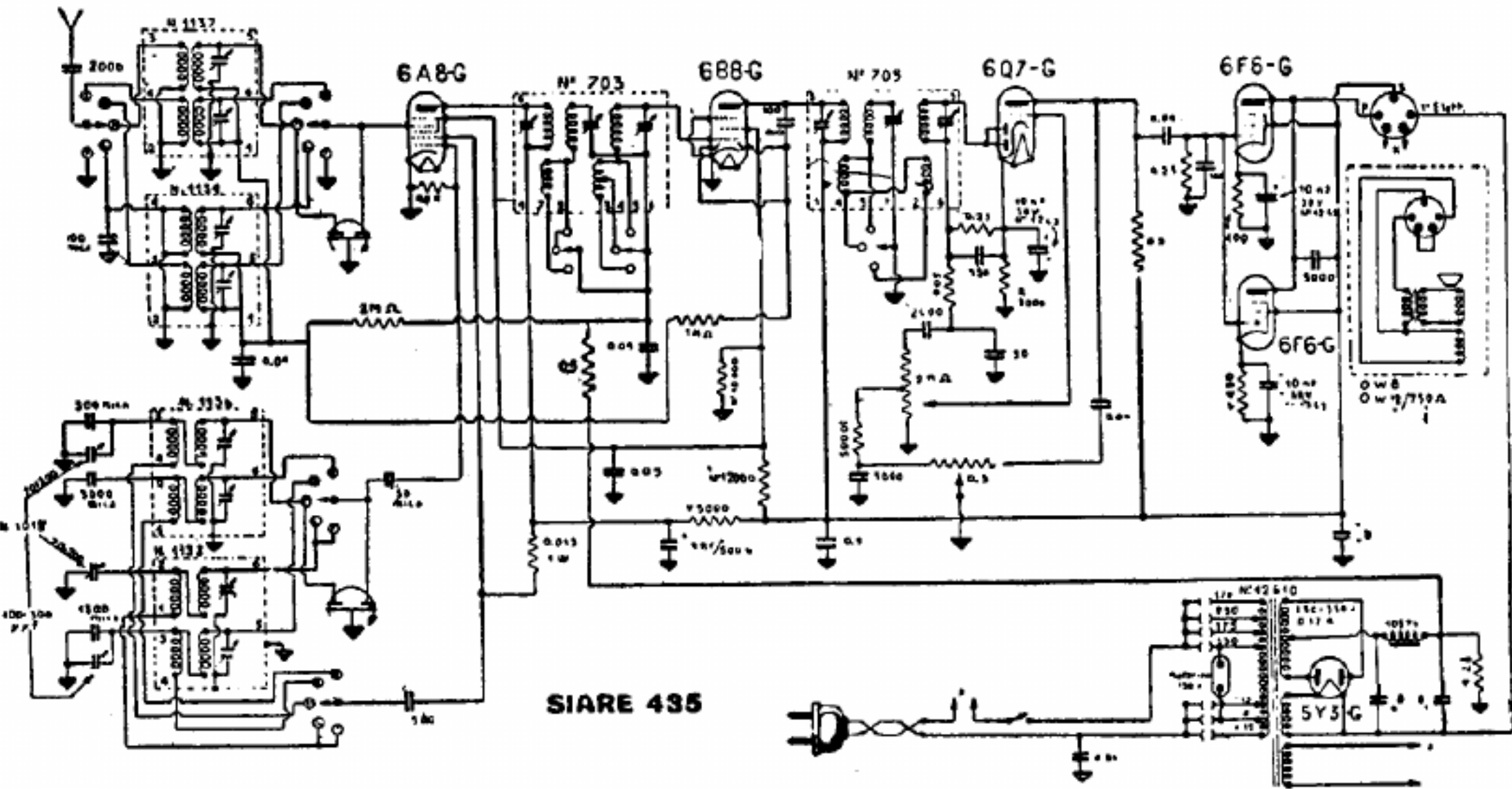
RADIO SIARE. — Mod. 435. — Produz 1938-39. — Gamme. cc. (17-27), c. (30-50), m. (210-520), l. (1200-1800). — Media frecuencia: 487 kHz.
